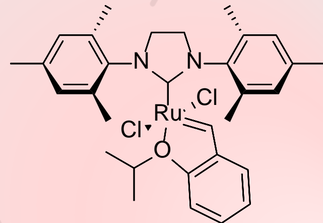
Hoveyda-Grubbs II
