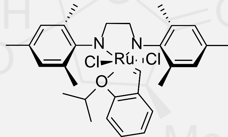
Hoveyda-Grubbs II
