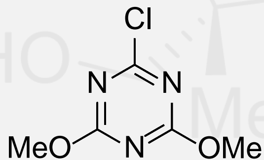
CDMT
