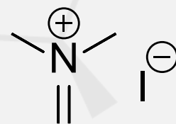
Eschenmoser's Salt
