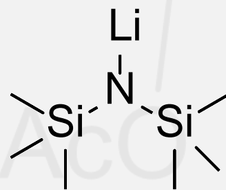
LiHMDS
