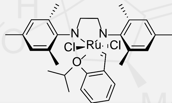
Hoveyda-Grubbs II
