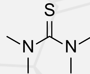
TMTU Tetramethylthiourea
