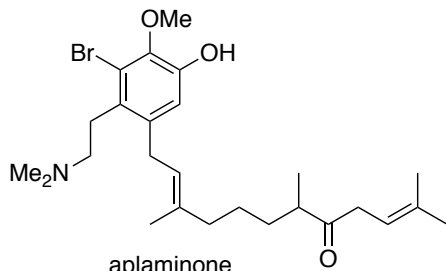
aplaminone
