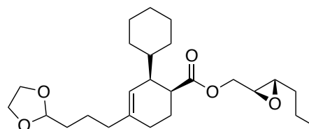
enantiomer shown
